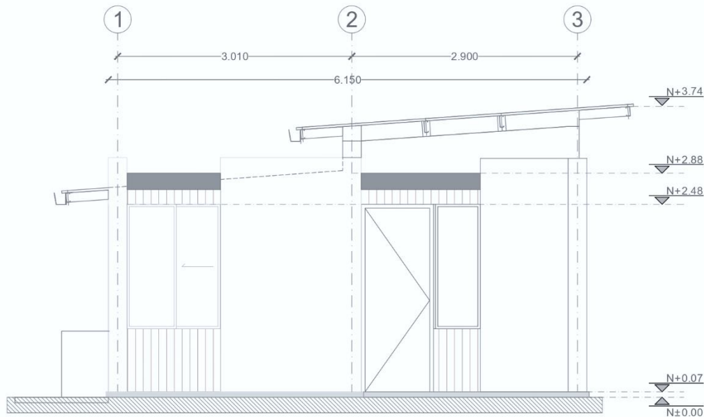
FACHADA FRONTAL
